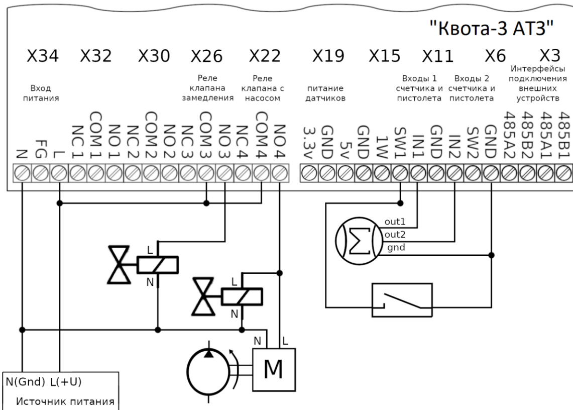
Рисунок 8: Схема подключения устройств в однопостовом режиме
