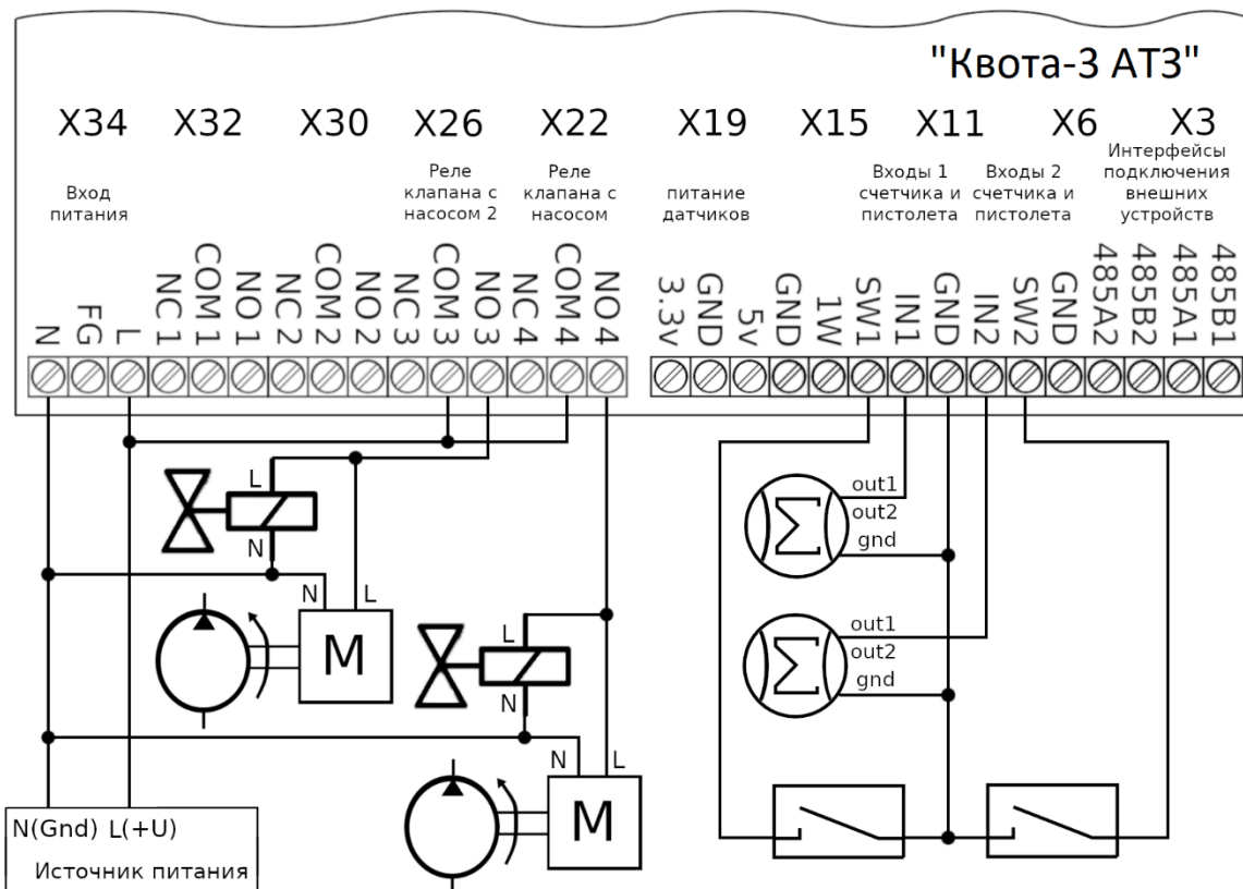
Рисунок 9: Схема подключения устройств в двухпостовом режиме
