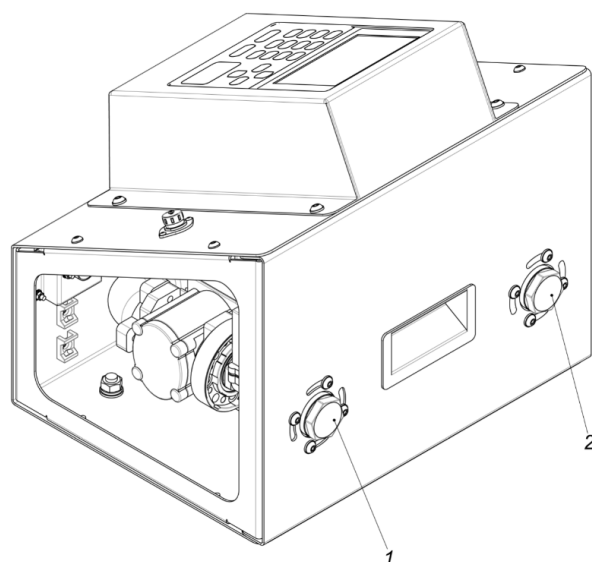
Рисунок 2. Тарировочная станция «ТС-752» (вид сзади): 1 – гидравлический выход из системы; 2 – гидравлический вход в систему
