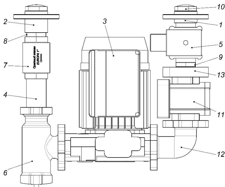
Рисунок 3. Гидравлическая система (вид сверху): 1 – фланец-переходник ВР 1” (выход); 2 – фланец ВР 1” (вход); 3 – насос; 4 – бочонок; 5 – электромагнитный клапан; 6 – линейный фильтр грубой очистки; 7 – обратный клапан; 8,9 – переходник-ниппель; 10 – пробка; 11 – импульсный счетчик; 12 – уголок; 13 – фланец
