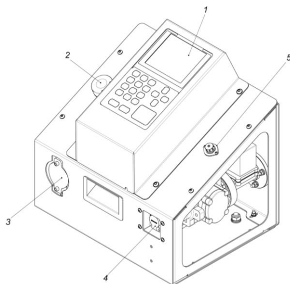
Рисунок 1. Тарифовочная станция «ТС-752» (вид спереди): 1 – контроллер «КБОТА-2»; 2 – антенна GSM-GPS; 3 – линейный фильтр грубой очистки; 4 – розетка USB; 5 – разъем для подключения ДУТ
