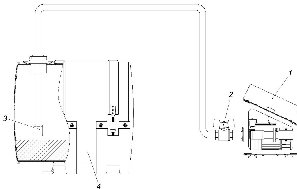
Рисунок 4. Схема подключения тарировочной станции к емкости (верхний забор топлива): 1 – тарировочная станция; 2 – шаровый кран; 3 – обратный клапан; 4 – резервуар
